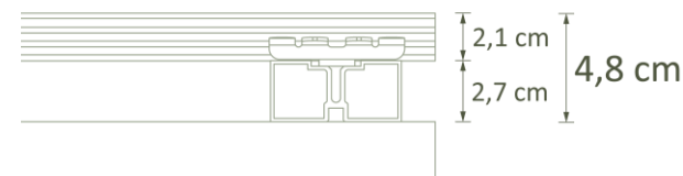
BARROTES EM ALUMÍNIO
